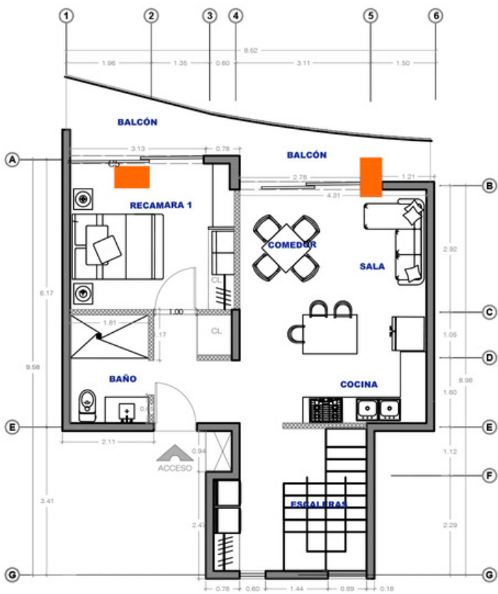
Planta Baja
