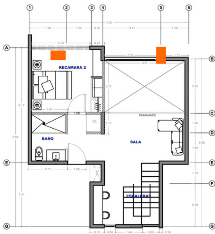
Planta Alta
